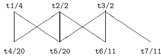
Obrázek 11: Precedence úloh
