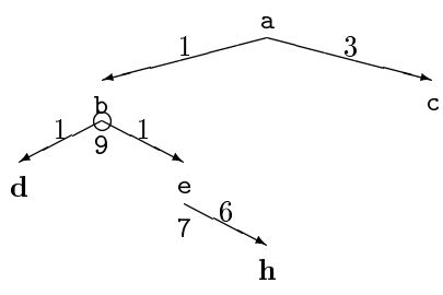
Obrázek 23: F(b)=9 > 3=F(c)
